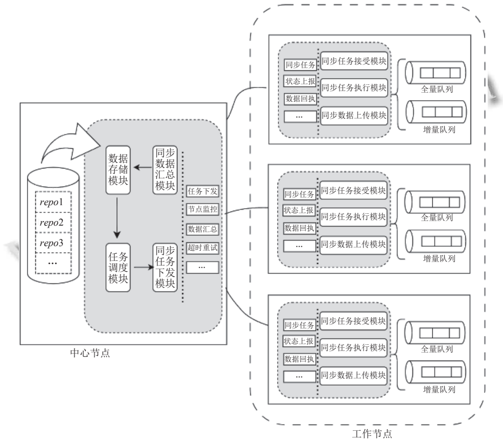
图 3 系统架构
