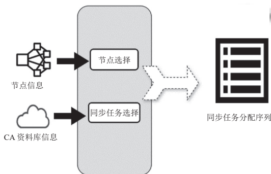
图4 任务调度
