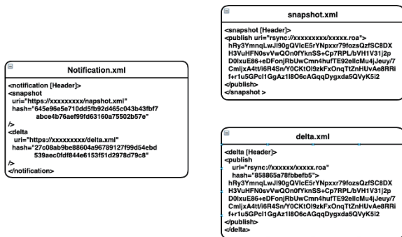
图1 通知文件
