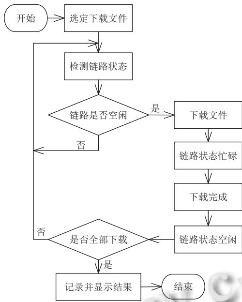
图4 单一链路下载流程图
