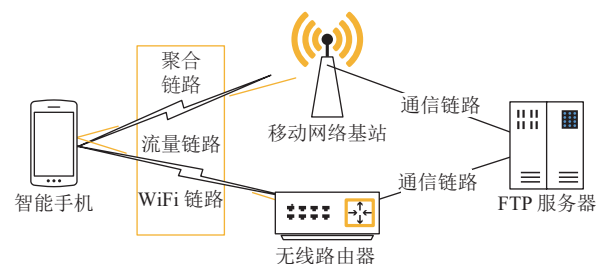
图 1 异构无线链路聚合示意图
