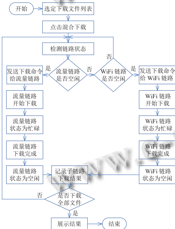
图5 聚合网络下载流程图
