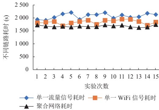
图 7 WiFi 信号较强环境下耗时统计
