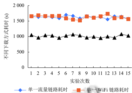
图 11 信号强度都比较强环境下耗时统计
