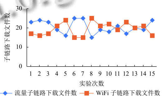
图 12 聚合网络子链路下载文件数
