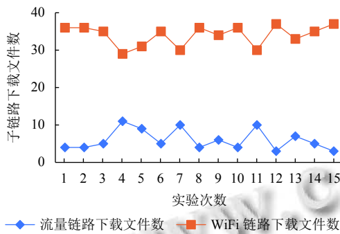
图 8 聚合网络子链路下载文件数目
