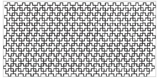
图9 十字型切割方案图(2000×1000)
