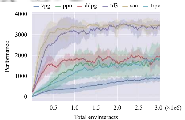
图 4 基于策略的强化学习算法(含 actor-critic)在 Hopper 问题的效果对比 [50]
