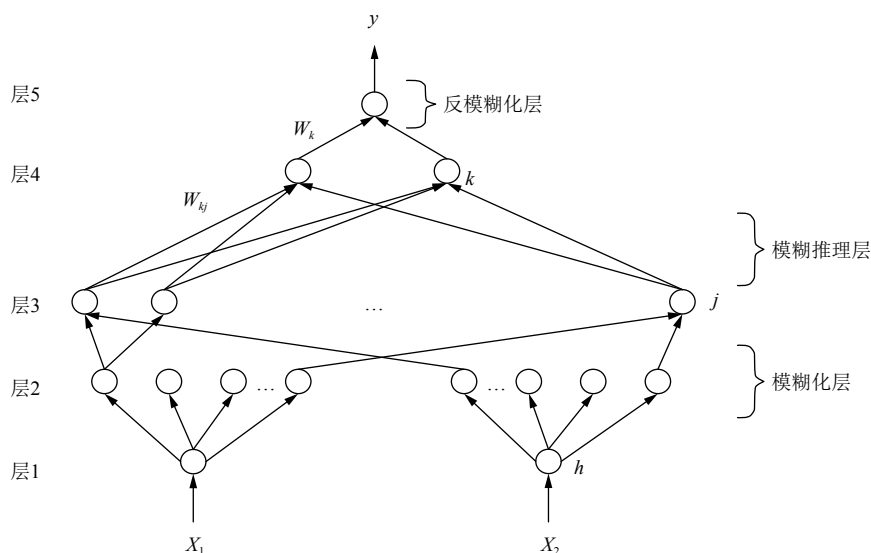
图1 传统模糊神经网络结构
