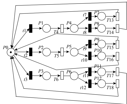
图 3 DDoS 攻防对抗网
