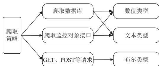
图 4 爬取策略
