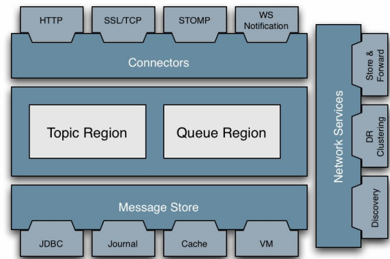
图 1 ActiveMQ 架构图
