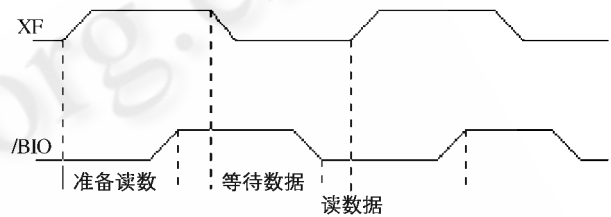
图 2 握手信号时序
