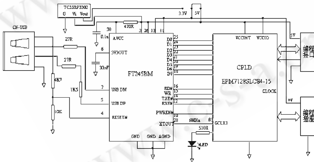
图 1 系统原理图
