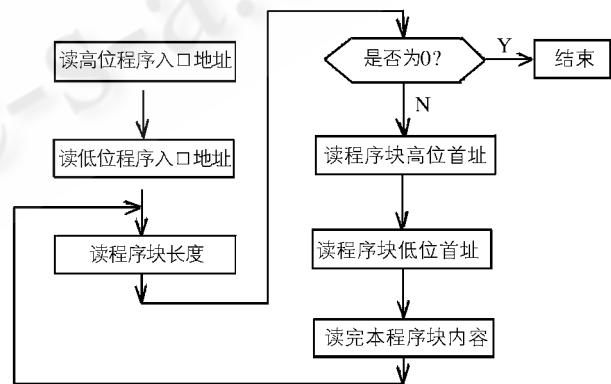
图 3 8 位并行 I/O Bootloader 程序框图
