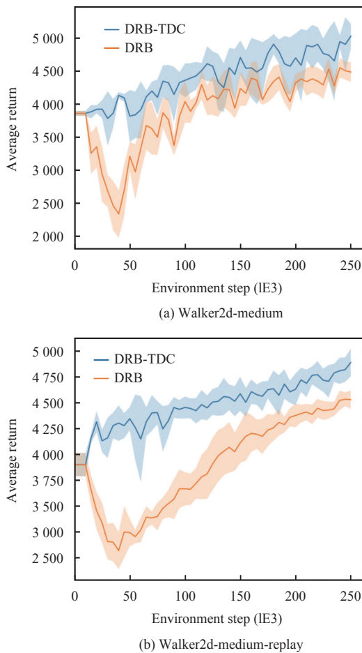
图 6 TDC 组件的消融实验
