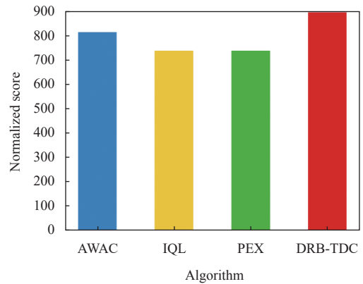
图4 所有任务的平均归一化得分总和
