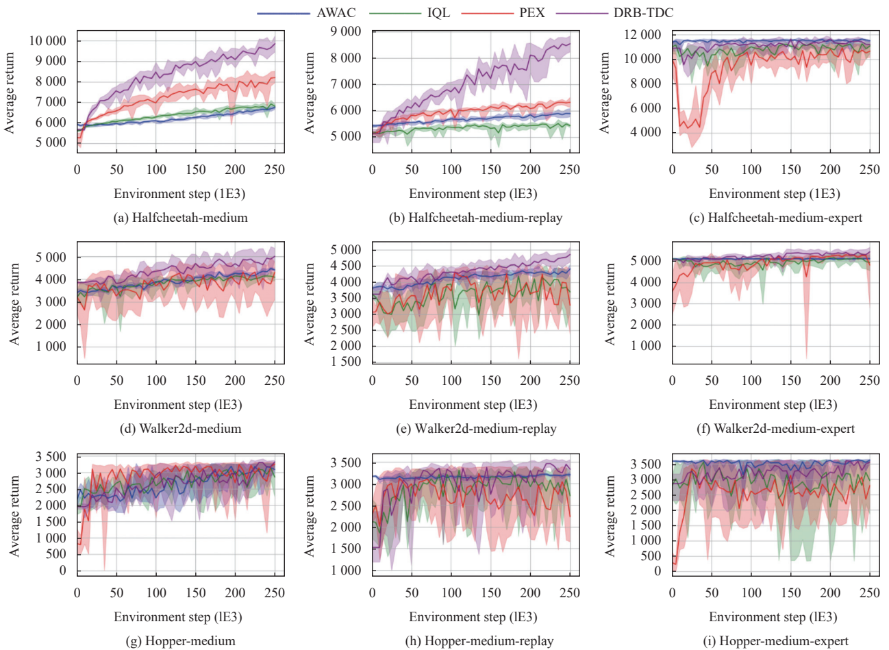
图 3 在线微调过程的策略性能评估
