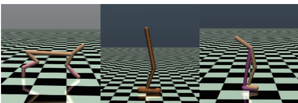
图 2 MuJoCo 环境
