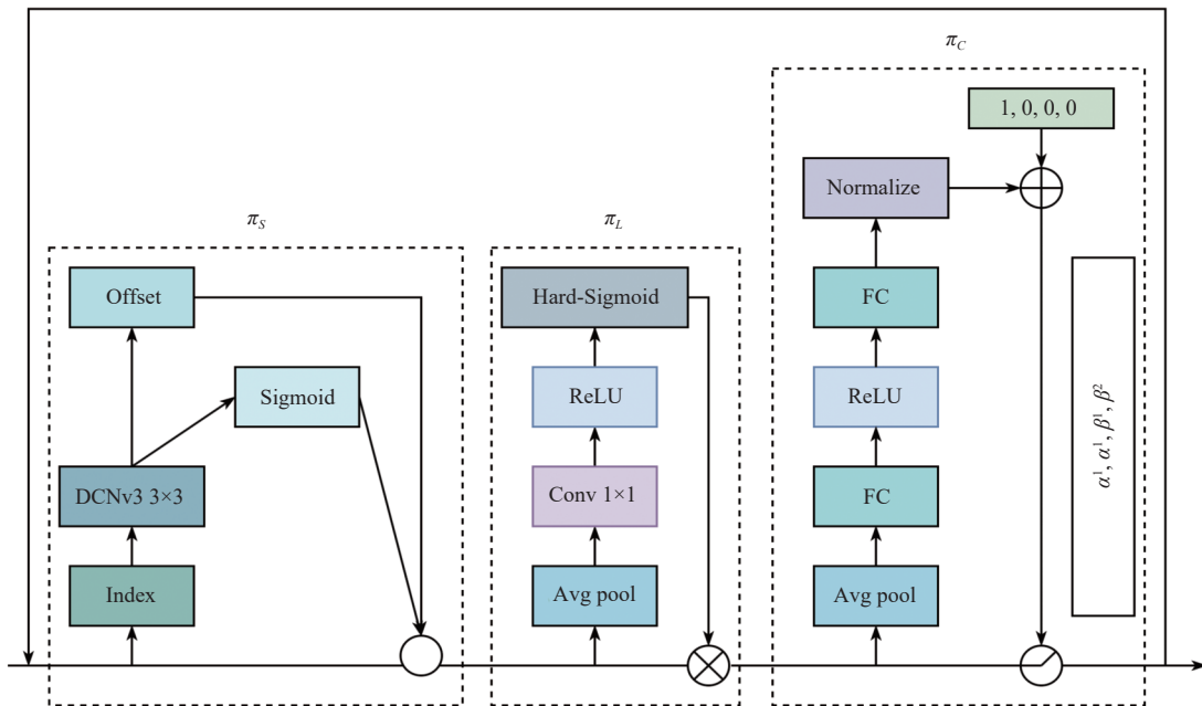
图4 改进动态头模块
