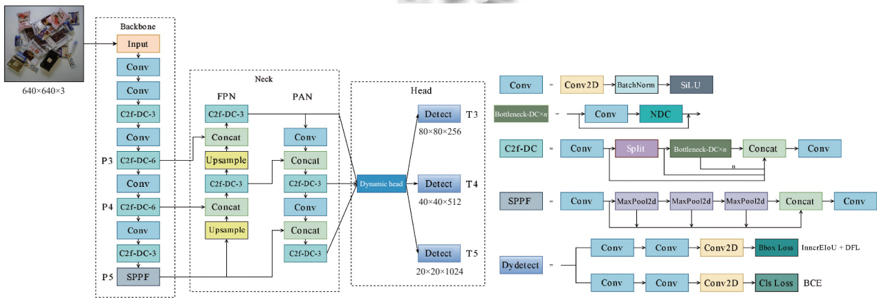
图1 YOLOv8-NDI的整体架构
