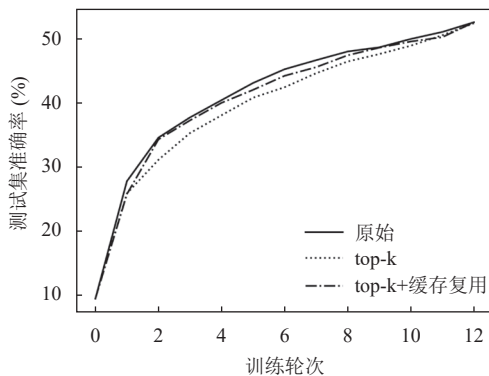
图 3 CIFAR10 数据集嵌入稀疏化测试结果
