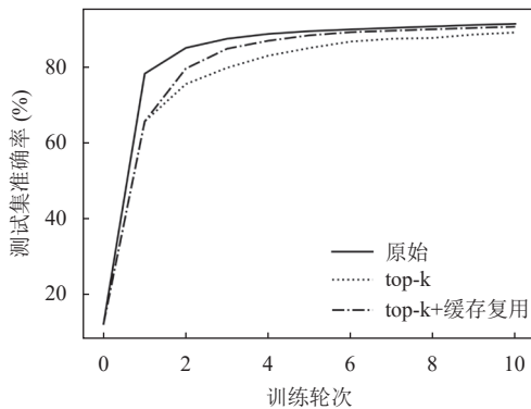
图 2 MNIST 数据集嵌入稀疏化测试结果
