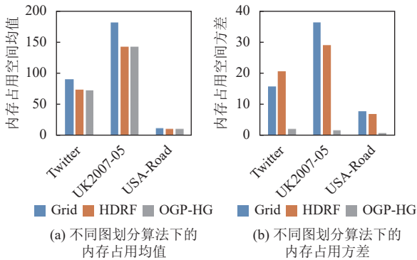
图 2 不同图划分算法下内存占用均值和方差
