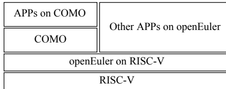
图 1 COMO 在 RISC-V 指令集和 openEuler 操作系统上的系统架构
