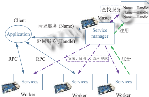
图4 COMO 技术的 ServiceManager 框架实现集群式 RISC-V 协同计算
