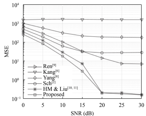
图 1 在 SUI 信道下不同定时算法的 MSE 对比
