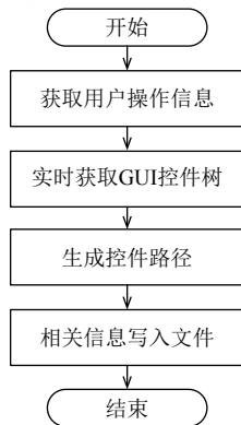
图2 跨设备脚本录制流程图
