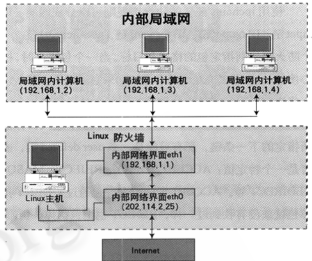
图 1 网络联接图
