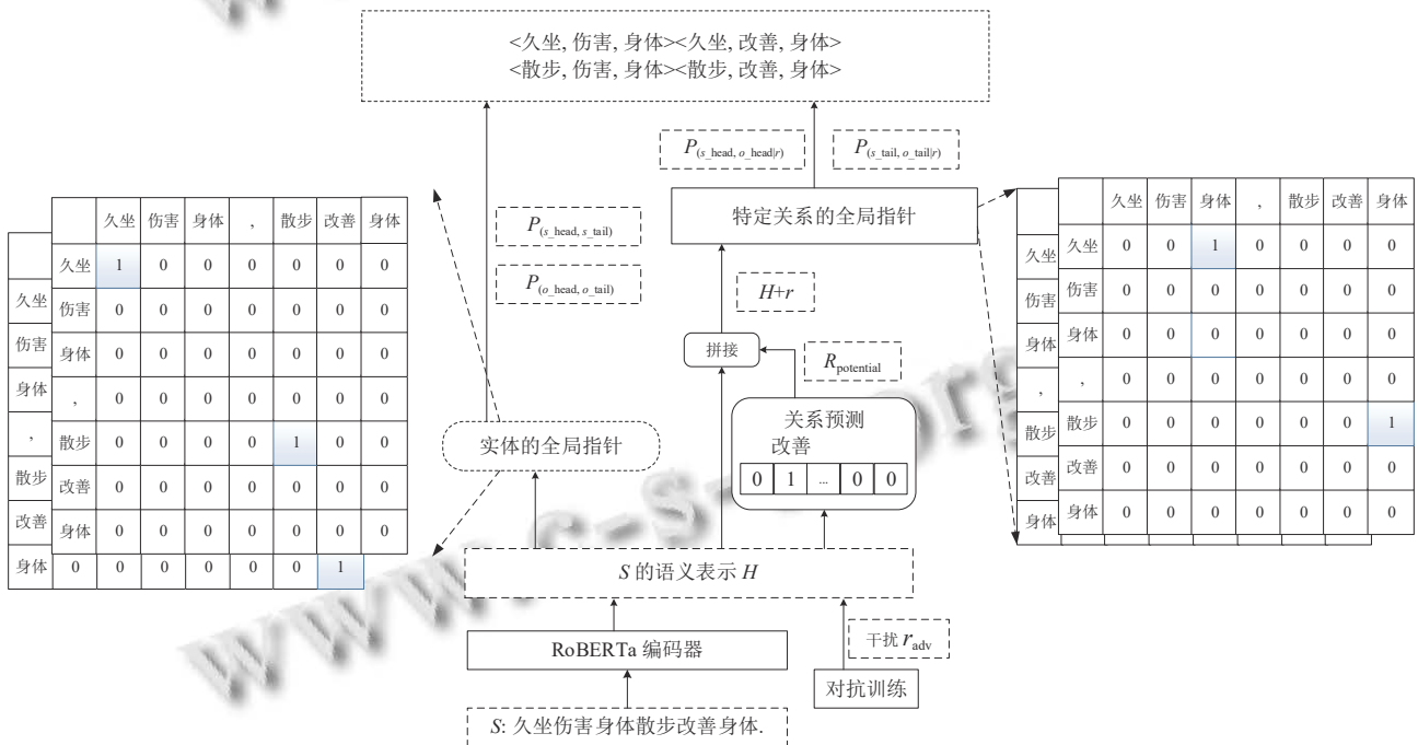
图 1 RGNRE 模型体系结构图
