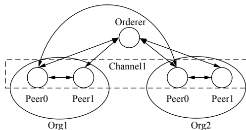
图 5 网络拓扑结构
