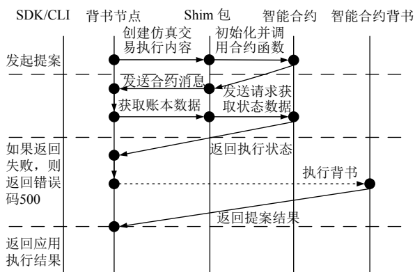
图 3 智能合约执行流程图
