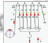
图 4 游车-天车-传动绞车系统分析计算模型
