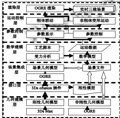
图 3 参数化油田钻井虚拟仿真系统开发框架
