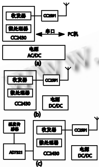
图 3 网络节点硬件框图
