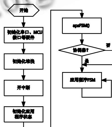
图 5 下位机系统程序流程图
