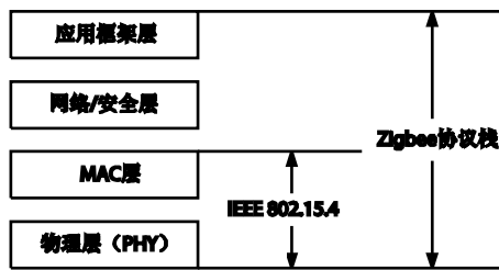
图 1 ZigBee 技术协议组成
