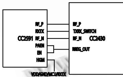
图 4 CC2591 与 CC2430 的接口
