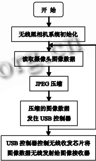
图 3 主程序流程图
