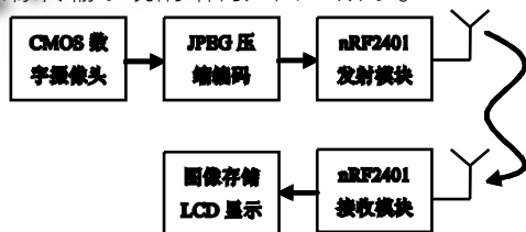
图 1 无线实时图像传输系统结构图
