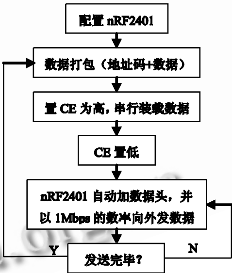
图 6 nRF2401 无线发送程序流程图
