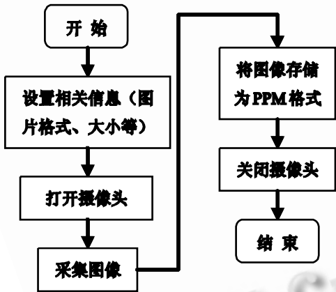
图 4 图像采集程序流程图
