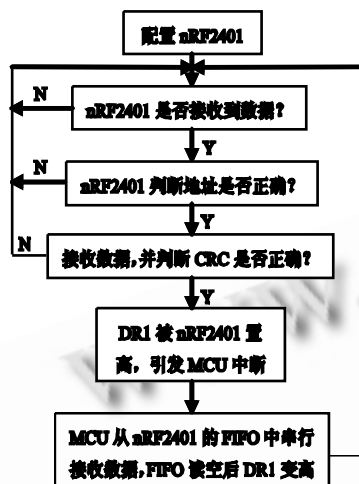
图 8 nRF2401 无线接收程序流程图
