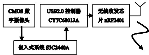
图 2 嵌入式无线照相机系统硬件结构
