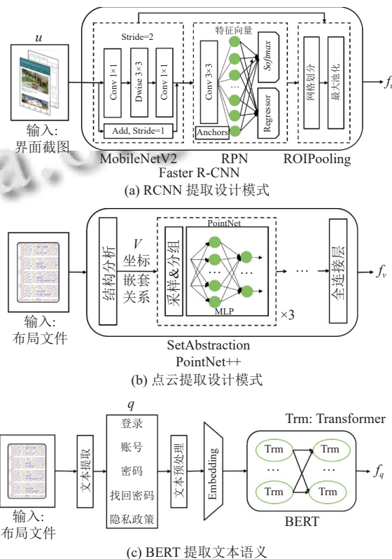
图5 特征提取示意图
