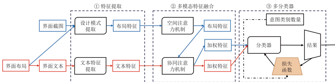
图4 用户意图识别模型结构
