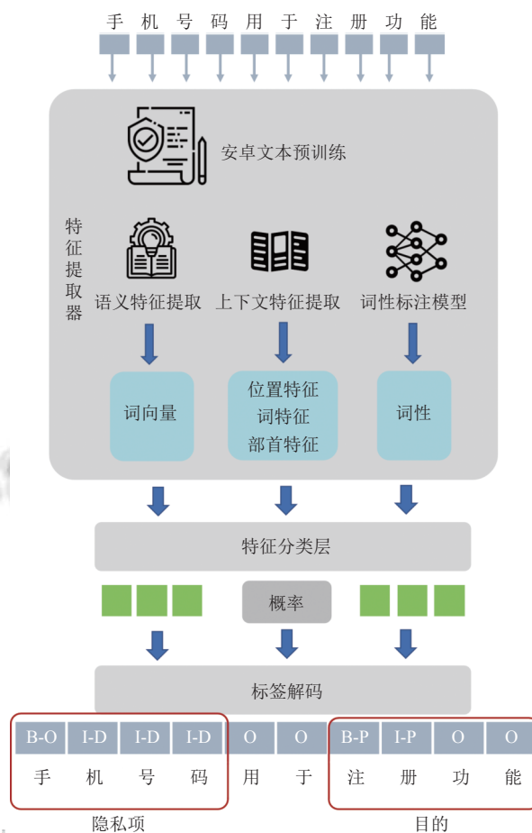
图 2 目的短语提取方法架构
