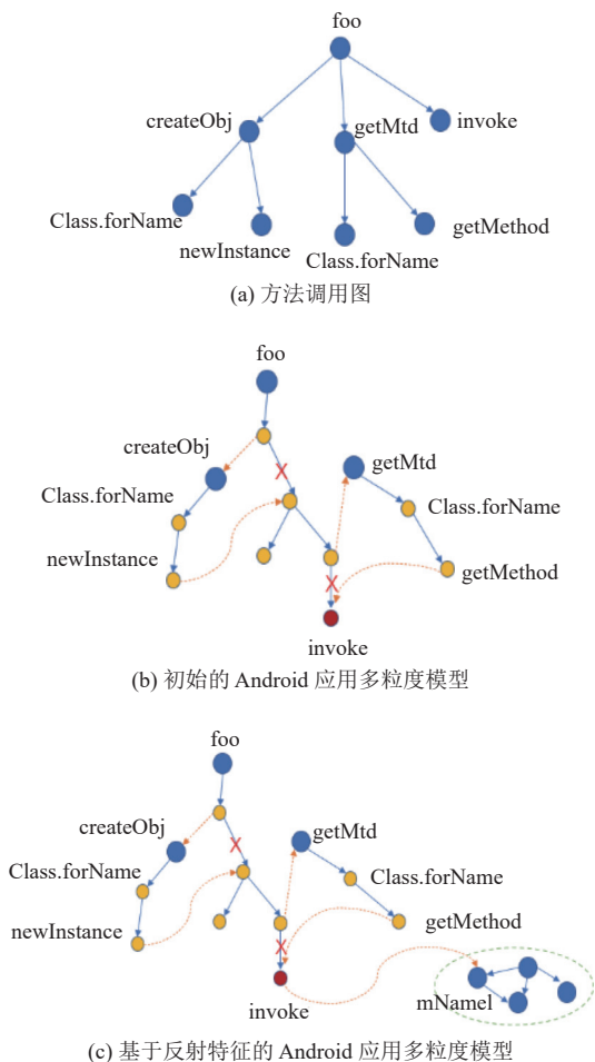
图 3 基于反射特征的 Android 应用多粒度模型构建过程
