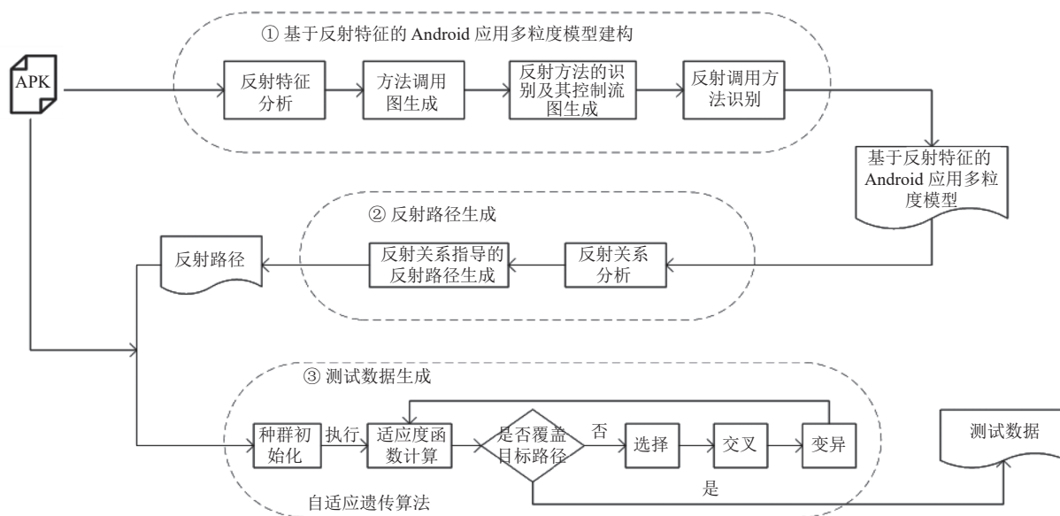
图 1 基于反射特征的 Android 测试用例自动生成方法框架
