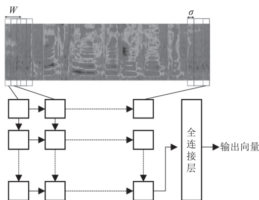
图7 LC-GRNN 工作流程
