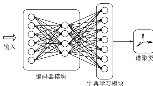
图 1 DNNDL 框架图
