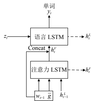
图 2 LSTM 模型图
