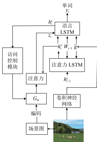
图 1 网络架构
