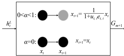
图 4 访问控制模块结点更新
