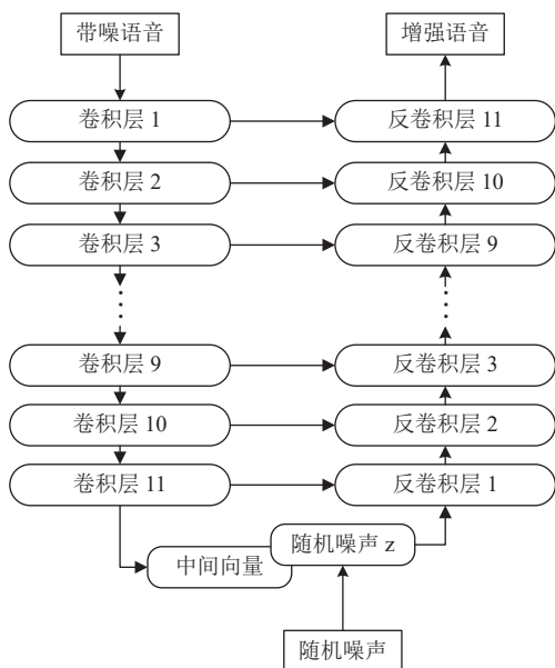
图2 SEGAN 的生成器
