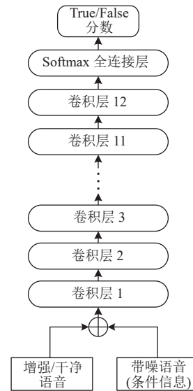
图3 SEGAN 的鉴别器
