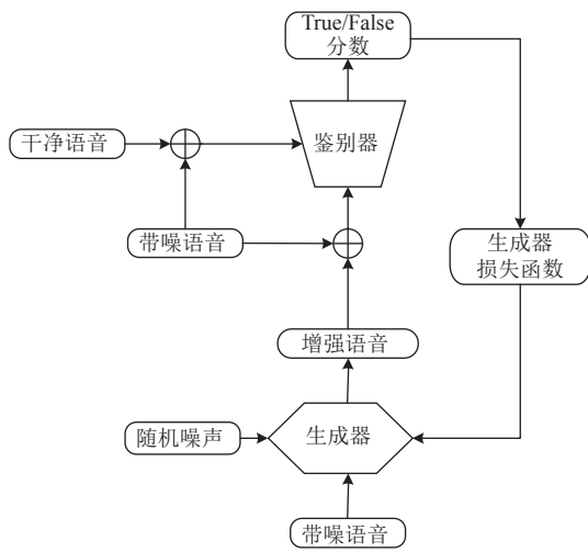
图1 SEGAN 模型框架
