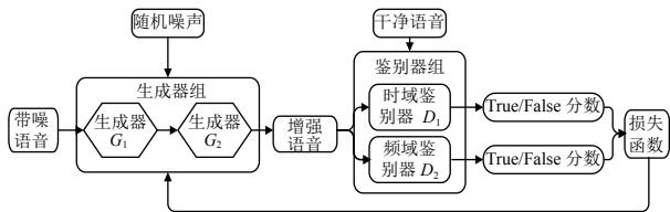
图 4 MS-TFSEGAN 模型框架
