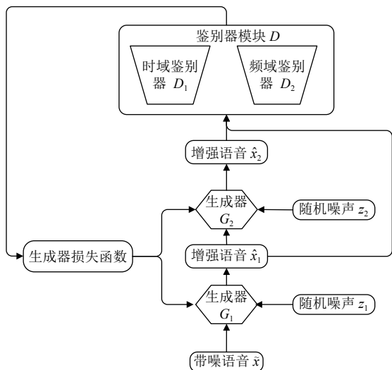
图 5 MS-TFSEGAN 的生成器
