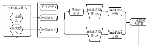
图 6 MS-TFSEGAN 的鉴别器框架
