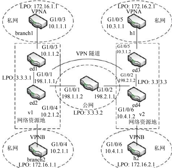
图2 采用网络设备虚拟化技术构建的网络拓扑
