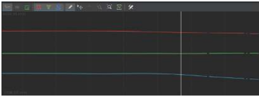
图6 动作帧面板
