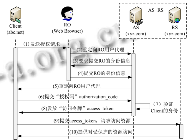
图 2 OAuth2.0 的跨域授权操作流程
