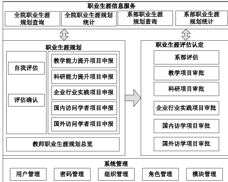
图 2 系统功能模型
