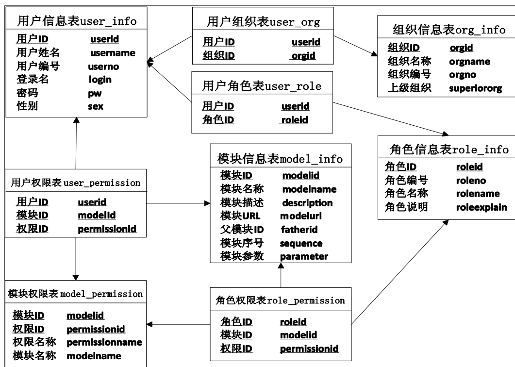
图 7 权限管理数据库设计
