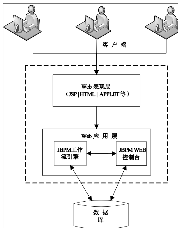
图 1 JBPM 在 WEB 容器中的运行架构图
