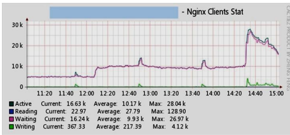
图 1 金山游戏官方网站 2009 年 nginx 集群连接数
