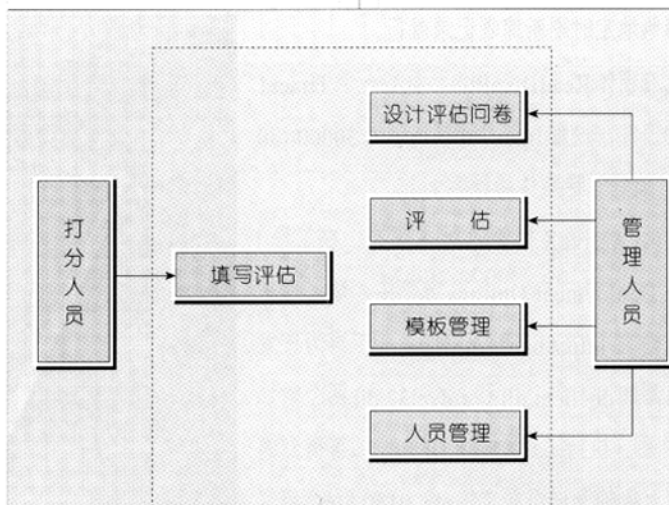
图 1 用例图
